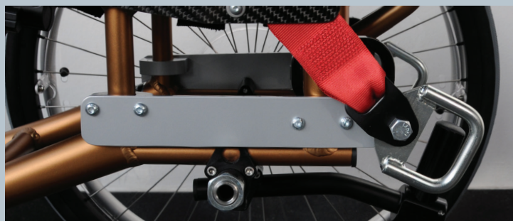
Zwei hintere Kraftknotensysteme mit jeweils einer genormten Schwerlastöse für Spannretraktor. Der Beckengurt ist bereits fest montiert.
